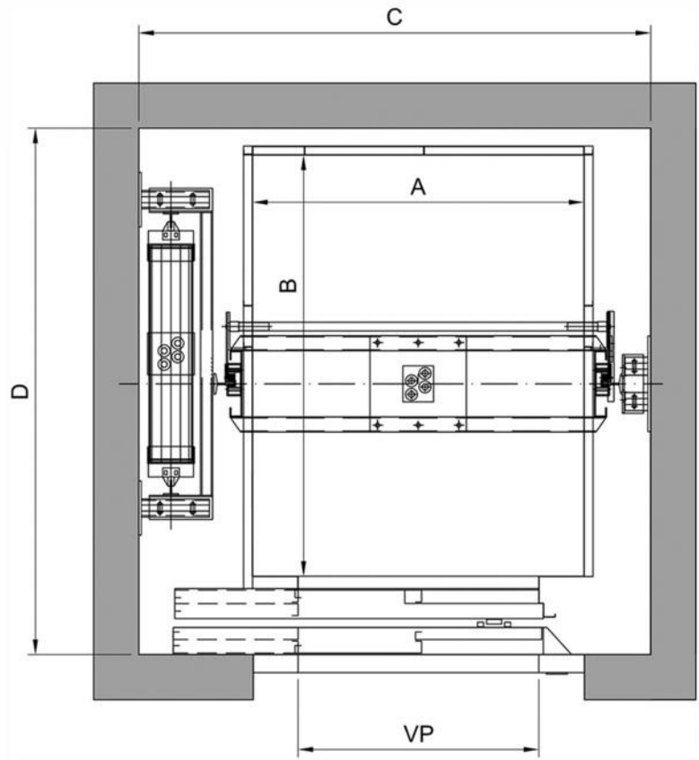
PLANTA BAIXA
